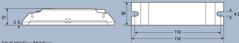
DALI® MULTleco/MULTleco
